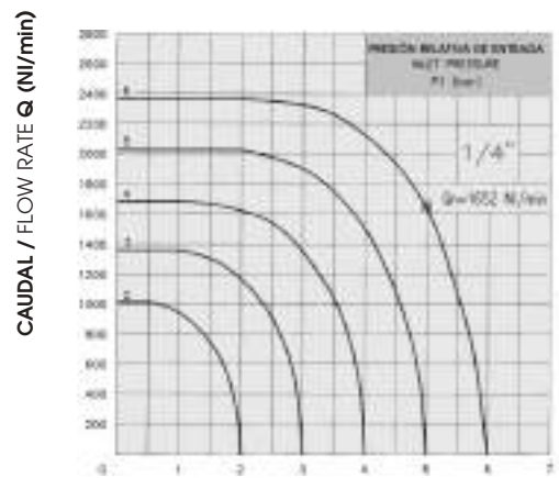
PRESIÓN RELATIVA SALIDA OUTLET PRESSURE P2 (bar)
