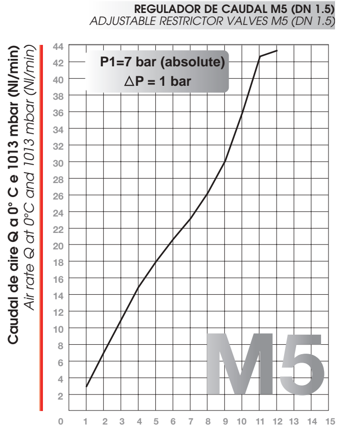
Número de giros tornillo regulador Number of turns of the adjusting needle
