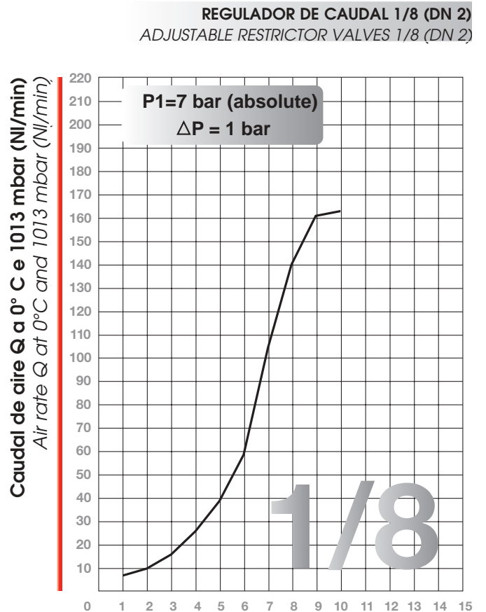
Número de giros tornillo regulador Number of turns of the adjusting needle
